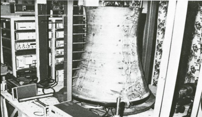
Model chłodni kominowej projektu Oswalda Matei
